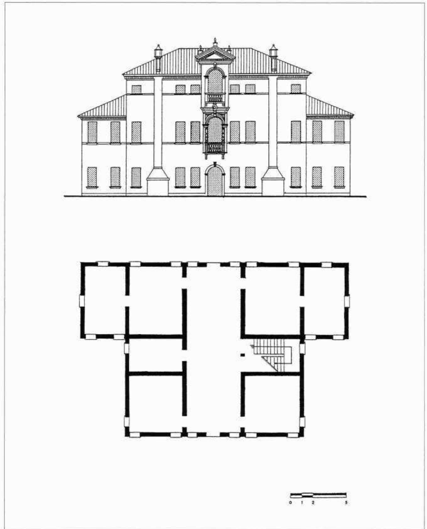
L'edificio residenziale: fronte meridionale e schema planimetrico del piano terreno
